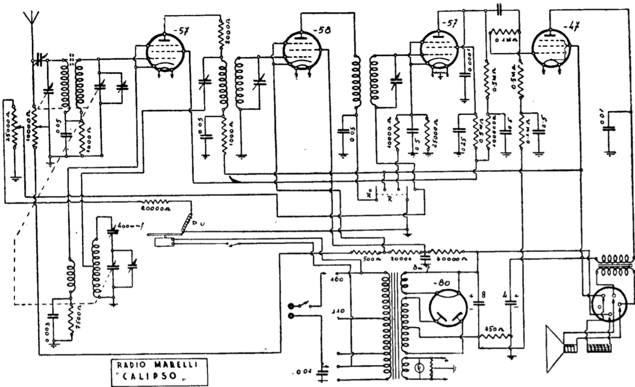
RADIO MARELLI. — Modello « Calipso ». - Produzione 1934 - Media frequenza: 175 kc.
